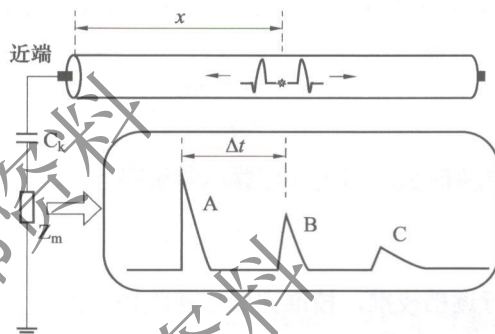
图 3 时域定位中局放脉冲反射示意图
