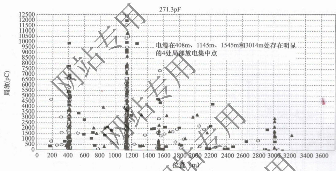
图 D.11 1.7U 0 局部放电点分布
