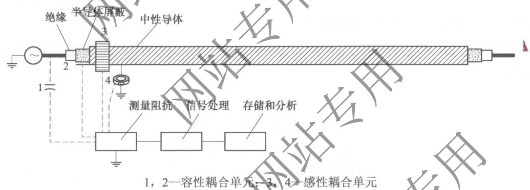
图 B.2 典型的局部放电测试系统
